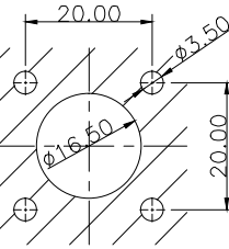
开孔尺寸
