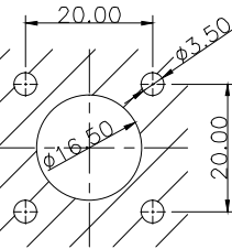
开孔尺寸
