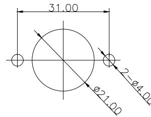
开孔尺寸
