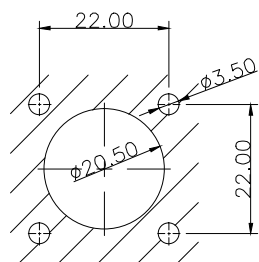
开孔尺寸
