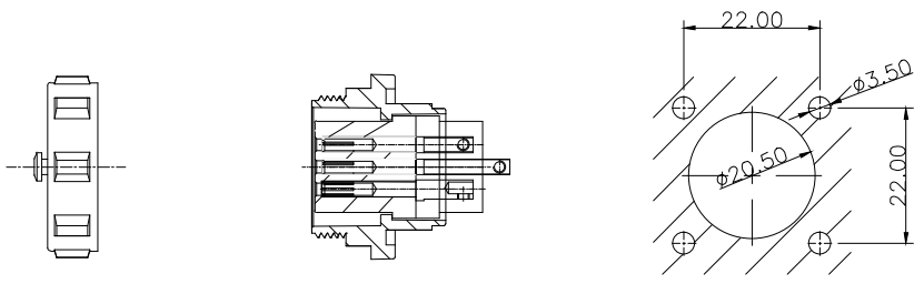
开孔尺寸
