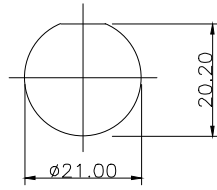
开孔尺寸 机箱板最厚3.0
